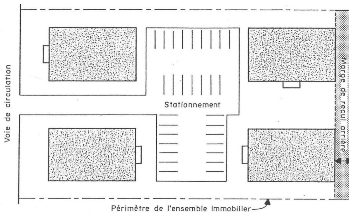
Figure III Marge de recul arrière
