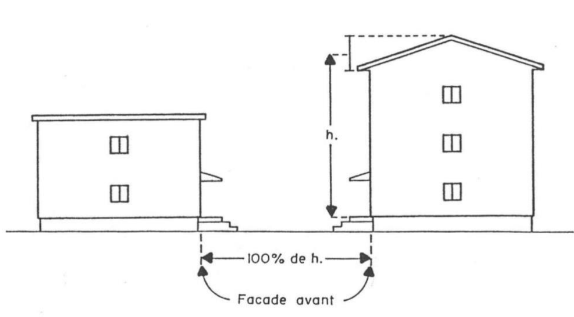
Figure IV Dégagement avant entre les bâtiments principaux
